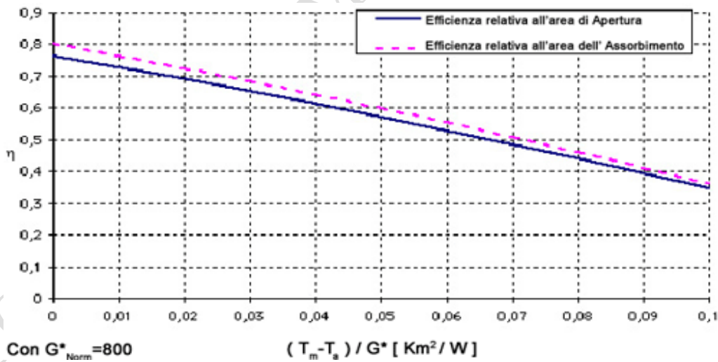
Grafico rendimento collettore solare
